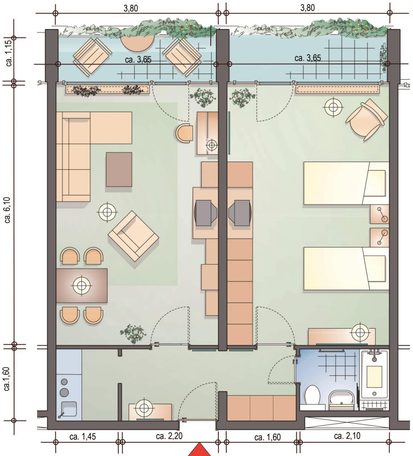
Zweizimmer-Wohnung Typ D6
